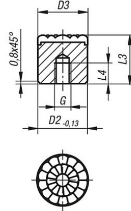
Forme P Insert en Inox à surface plate rectifiée et surface polyuréthane
